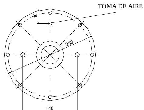
PLACA INFERIOR
